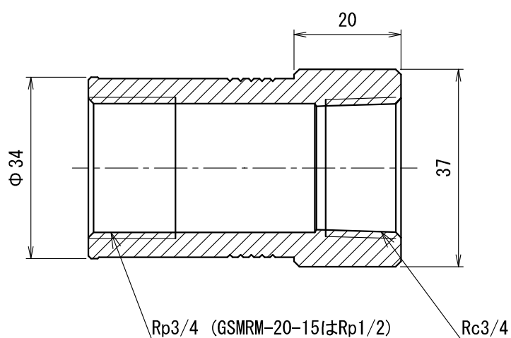
断面 A-A
